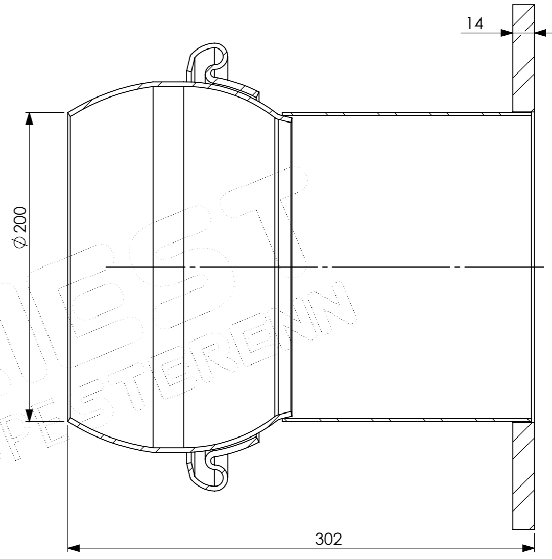
COUPE A-A
